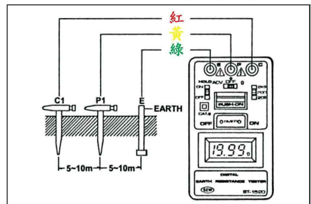
接地電阻量測接線圖
