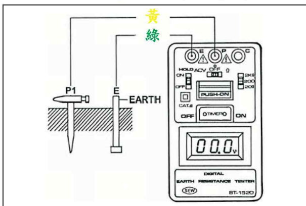
接地電壓量測接線圖
