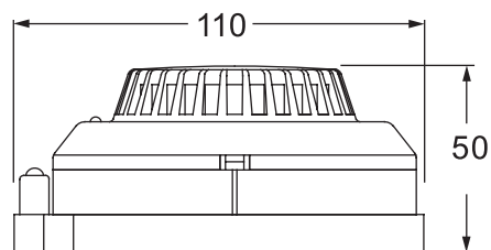
尺寸圖
